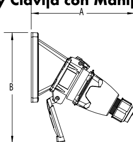
Tomacorriente en Ángulo de 30° y Clavija con Manija
