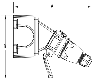
Tomacorriente con ángulo de 30° en Caja de Conexiones y Clavija con Manija
