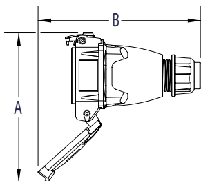
Tomacorriente con Manija
